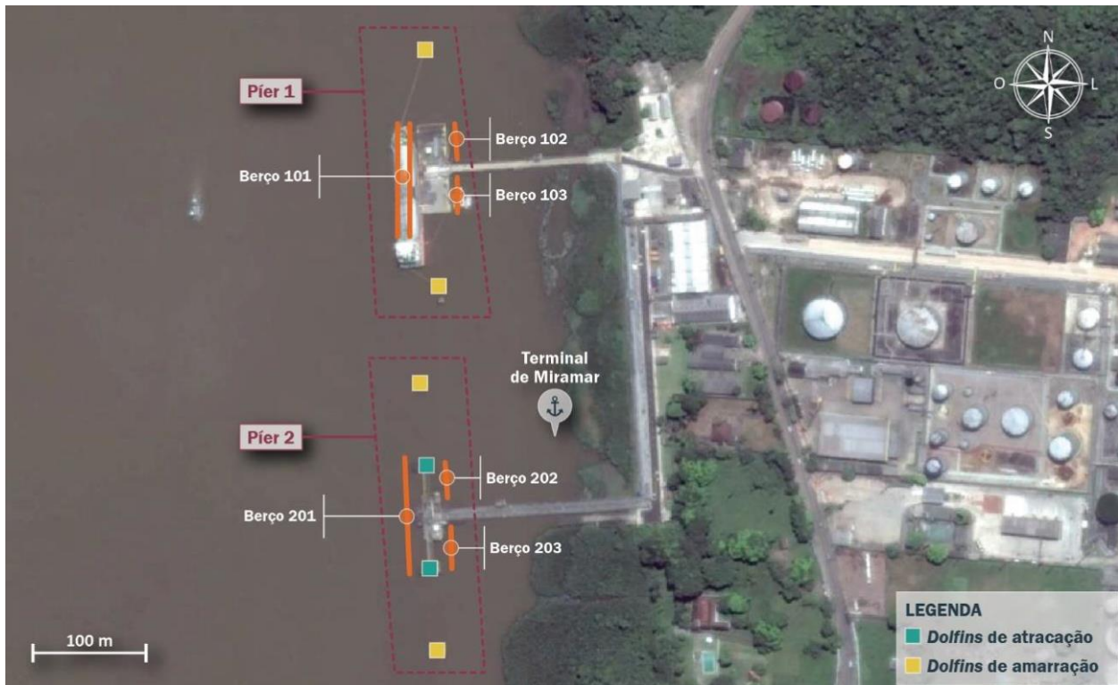
Figura 2: Infraestrutura de acostagem do Terminal Petroquímico de Miramar Fonte: Plano Mestre do Complexo Portuário de Belém e Vila do Conde (2017)
